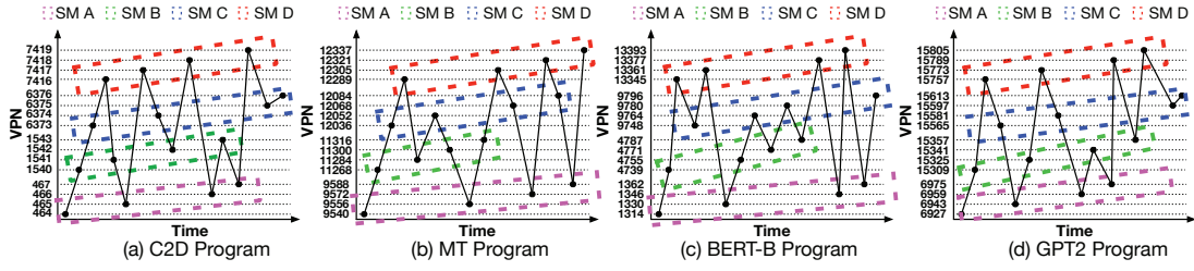
Fig. 3. Four SMs' access patterns of (a) C2D, (b) MT, (c) BERT-B and (d) GPT2
