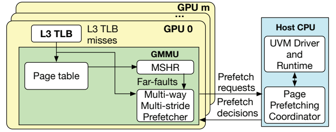
Fig. 7. LIBRA overview
